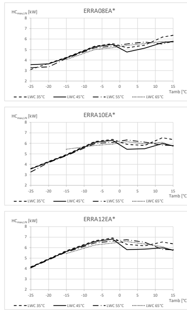
Capacità di riscaldamento massima - valori di picco
