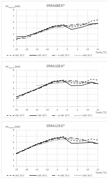
Capacità di riscaldamento massima - valore integrato
