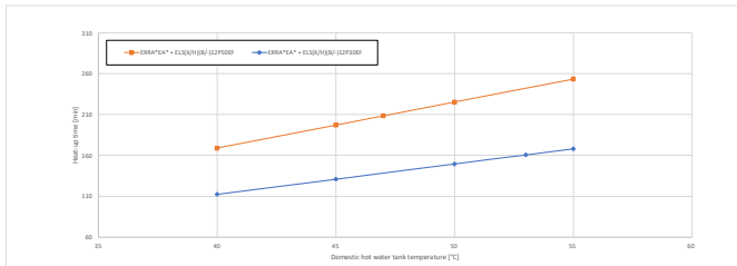
Tempi di riscaldamento
